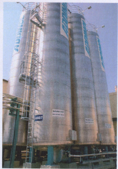
Im Außenbereich setzen die silbernen Tanks Akzente. Zur Lagerung von Grundölen und flüssigen Additiven stehen in den Hallen und außen 57 Tanks bereit.
